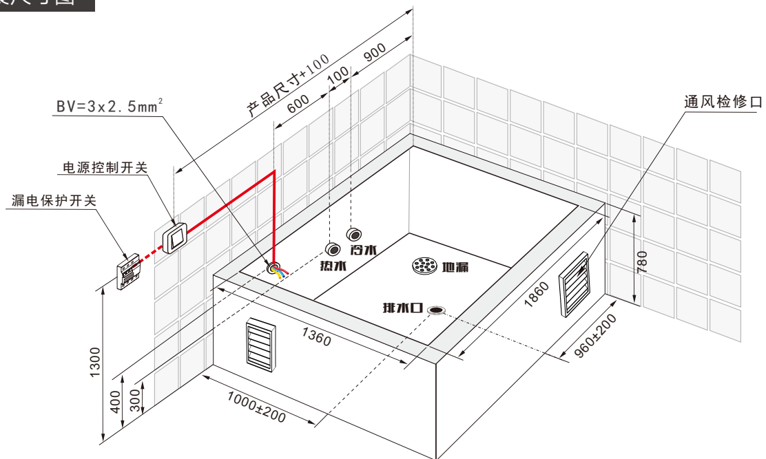
水电安装尺寸图
